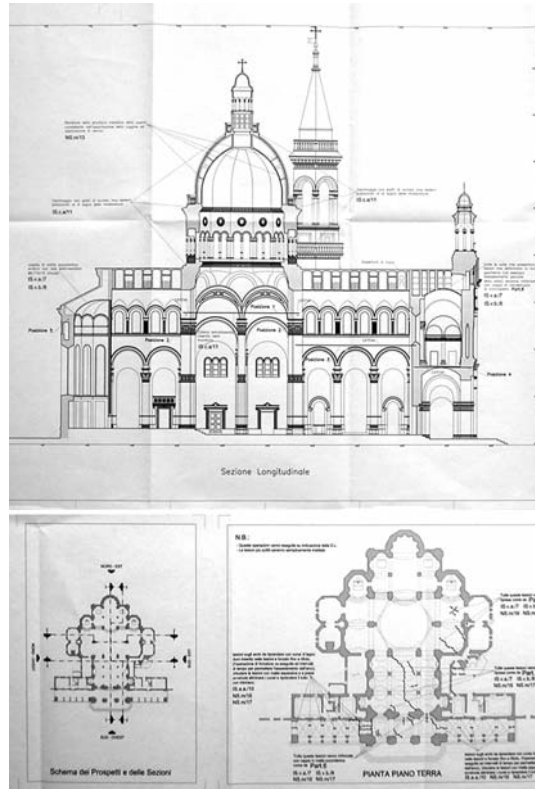
Particolari del progetto di costruzione del Santuario redatti dall'Arch. Costantino Costantini nel 1892
